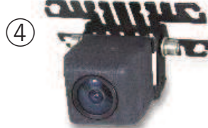
④ ミニキュブ広角型 WTJ636Fカメラ 水平147° 垂直80°
